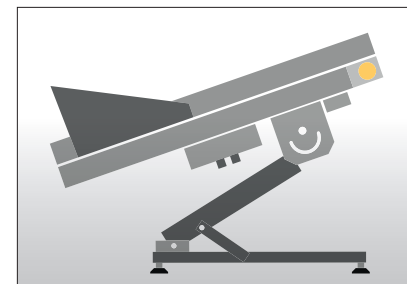
Über einen manuellen Kurbetrieb lässt sich die Höhe des Scherenfußes anpassen.
