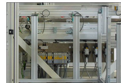
Druckluftkomponenten.
